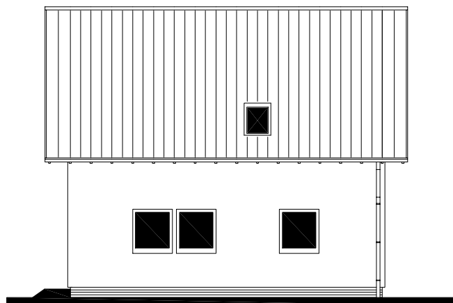
POHLED ZADNÍ
