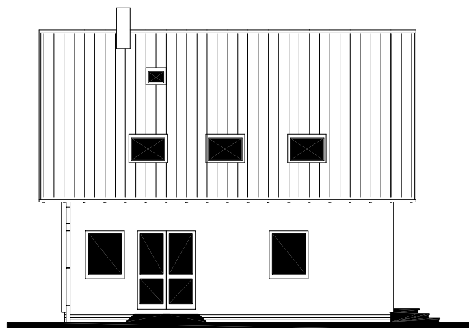
POHLED ZADNÍ
