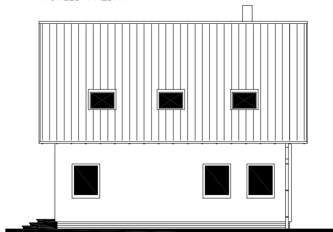
POHLED PŘEDNÍ
