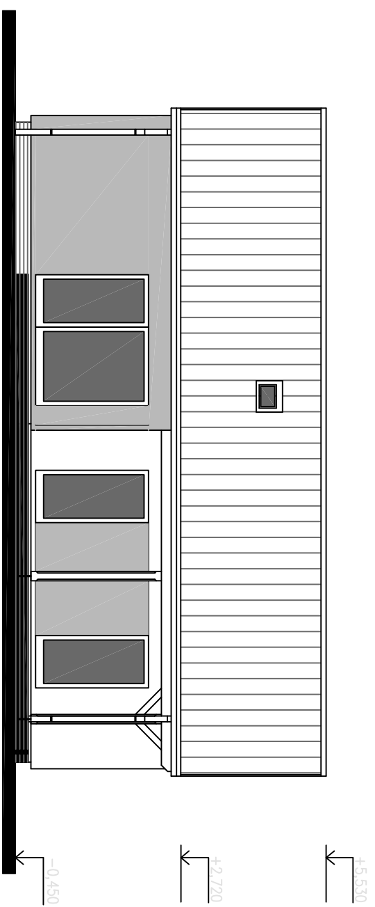
POHLED JIŽNÍ
